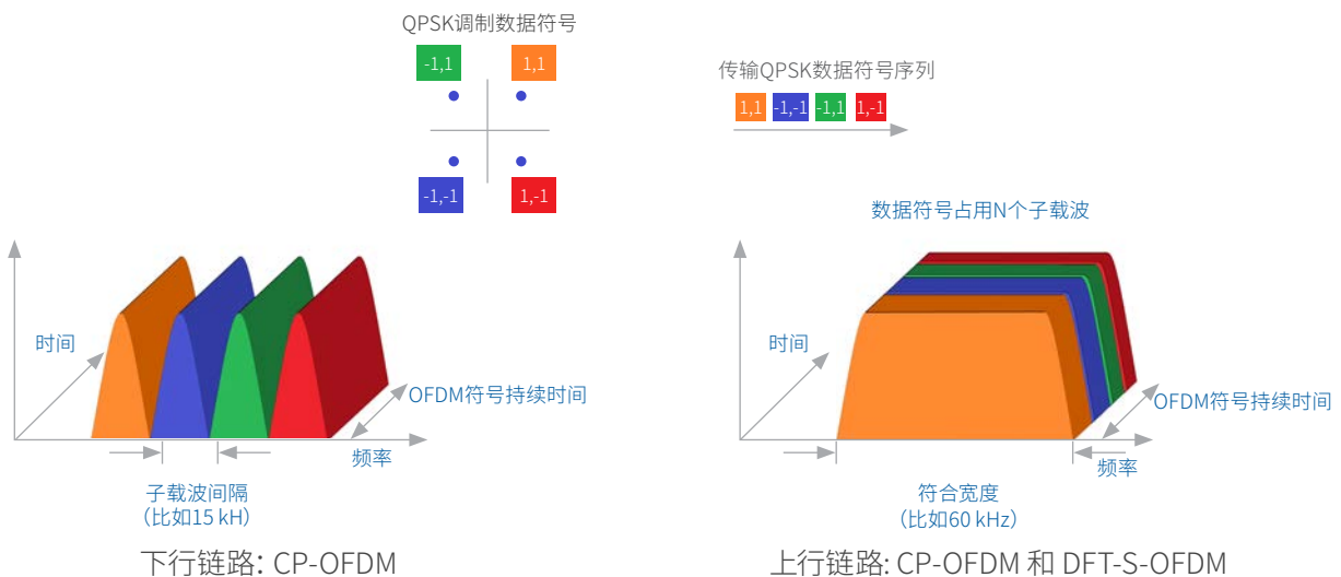
图5. OFDM与DFT-S-OFDM
